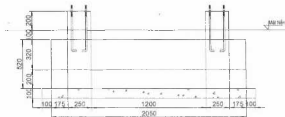
MẶT ĐỪNG DỌC
