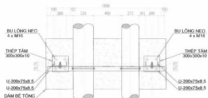
MẶT BẰNG CHI TIẾT GÓI ĐỖ
