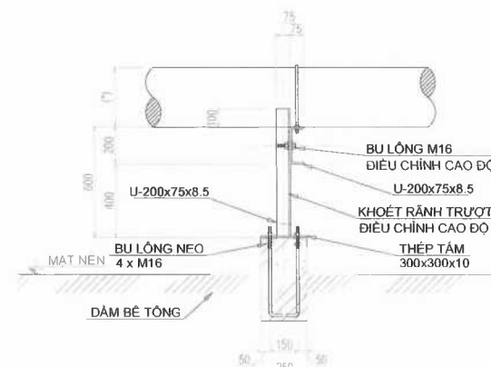
MẶT CẮT 2-2
