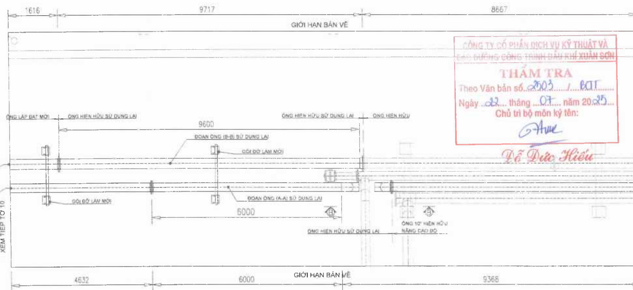
MẶT BẰNG ỐNG CẢI TẠO
