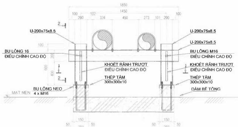
MẶT ĐỪNG CHI TIẾT GÓI ĐỖ SỐ LƯỢNG: 6 BỘ
