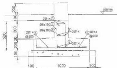
MẶT CẮT 1-1
