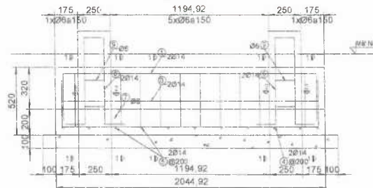
MẶT BẰNG BỐ TRÍ THÉP
