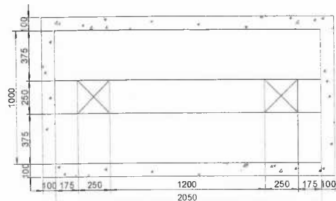
MẶT BẰNG MÓNG
