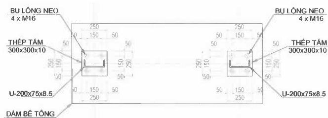
MẶT CẮT 1-1
