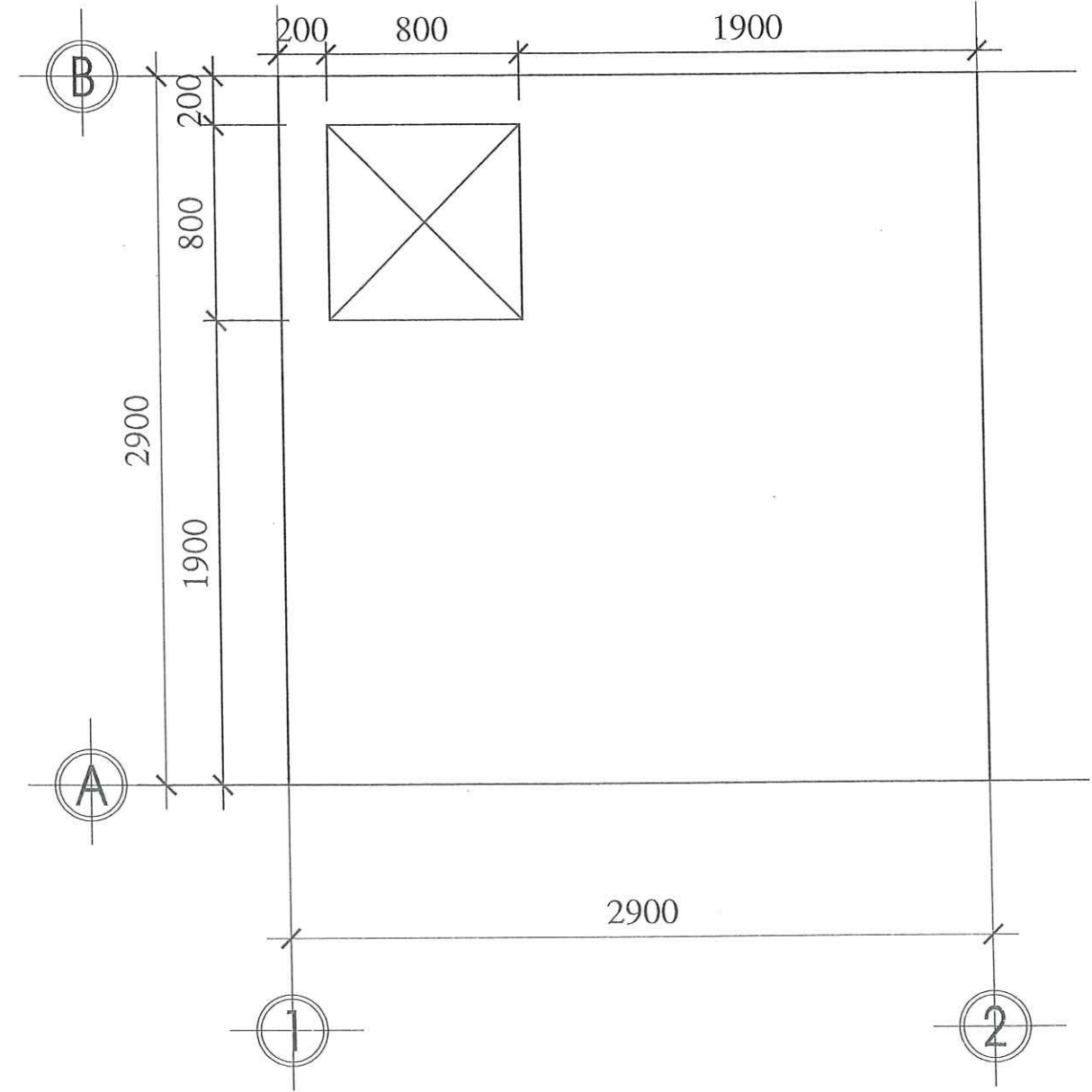
MẶT BẰNG BẢN NẮP BỂ ĐIỀU HOÀ TL 1/100
