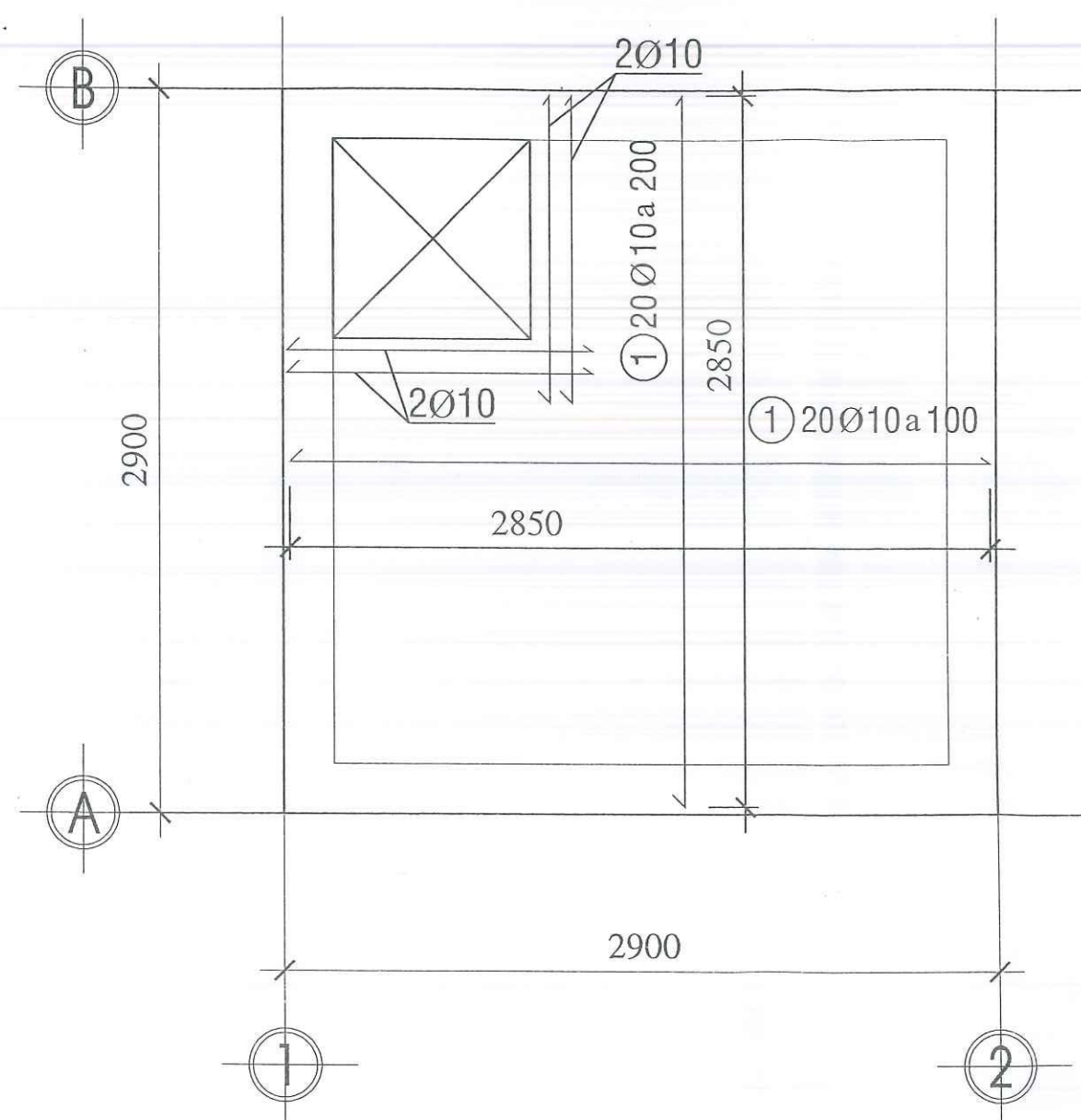
MẶT BẰNG BỐ TRÍ THÉP BẢN NẮP BỂ ĐIỀU HOÀ TL 1/100
