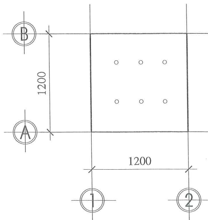
MẶT BẰNG BẢN NẮP HỒ GA TL 1/100
