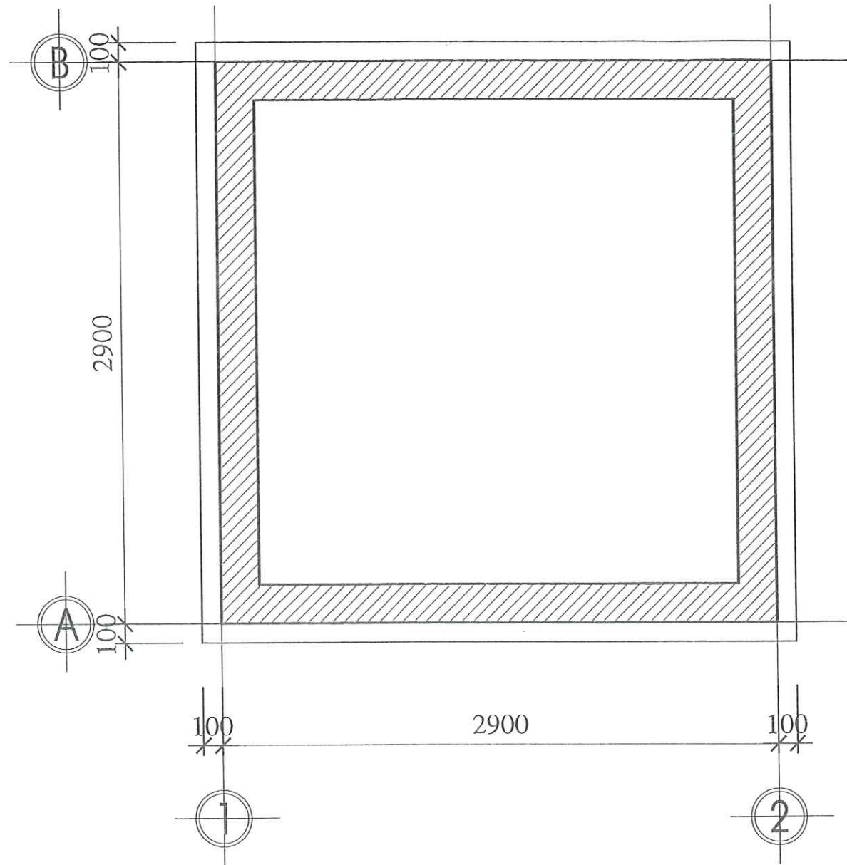
MẶT BẰNG BẢN ĐÁY BỂ ĐIỀU HOÀ TL 1/100
