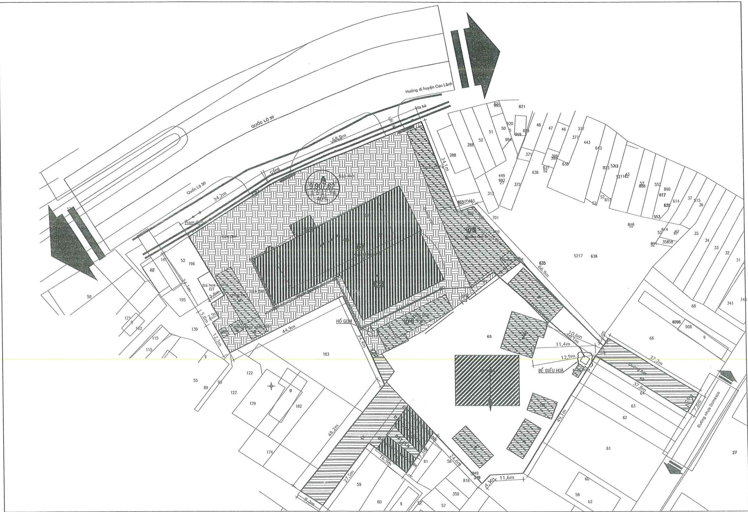
MẶT BẰNG VỊ TRÍ XÂY DỰNG TL 1/400
