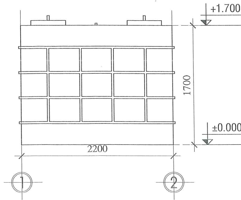
MẶT ĐỨNG TRỤC 1-2 TL 1/100
