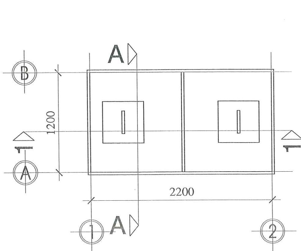
MẶT BẰNG BỒN NƯỚC TL 1/100
