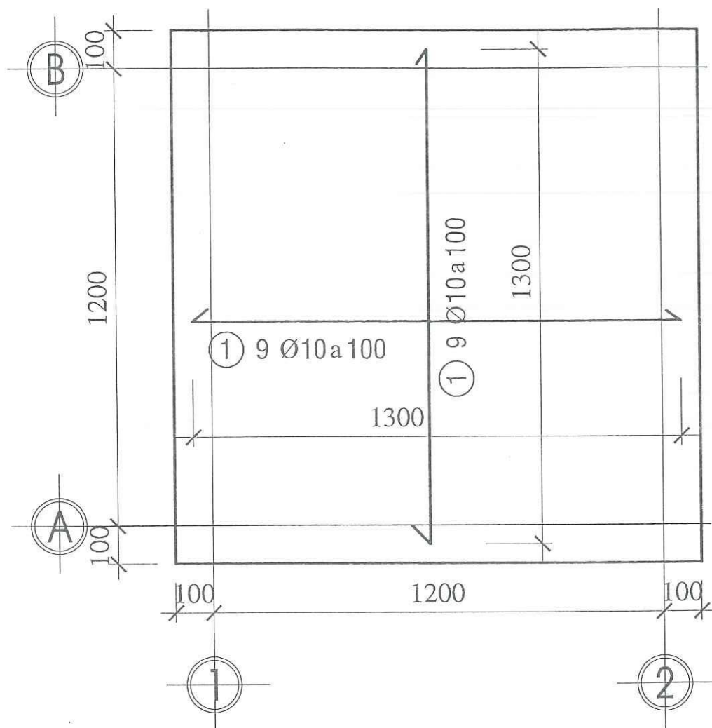
MẶT BẰNG BỐ TRÍ THÉP BẢN ĐÁY BỂ ĐIỀU HOÀ TL 1/100
