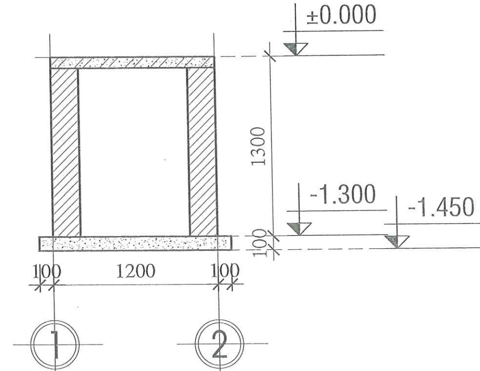
MẶT CẮT 1-1 BỂ ĐIỀU HOÀ TL 1/100
