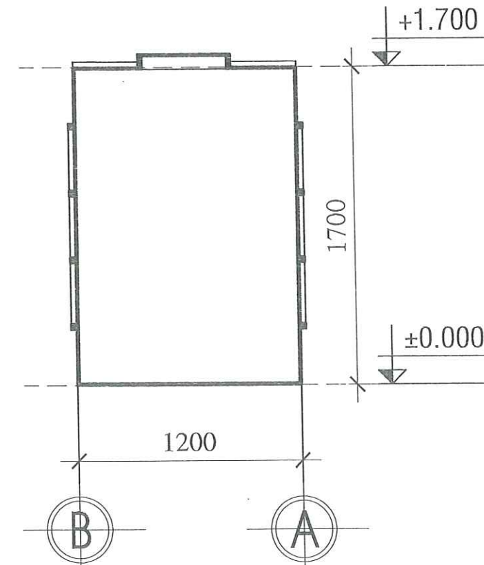
MẶT CẮT A-A TL 1/100
