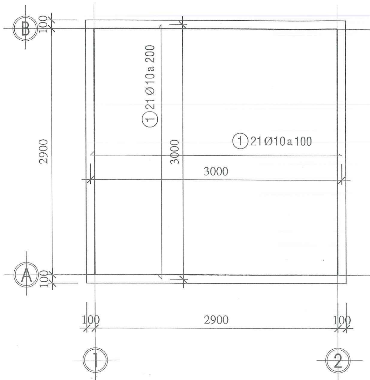
MẶT BẰNG BỐ TRÍ THÉP BẢN ĐÁY BỂ ĐIỀU HOÀ TL 1/100
