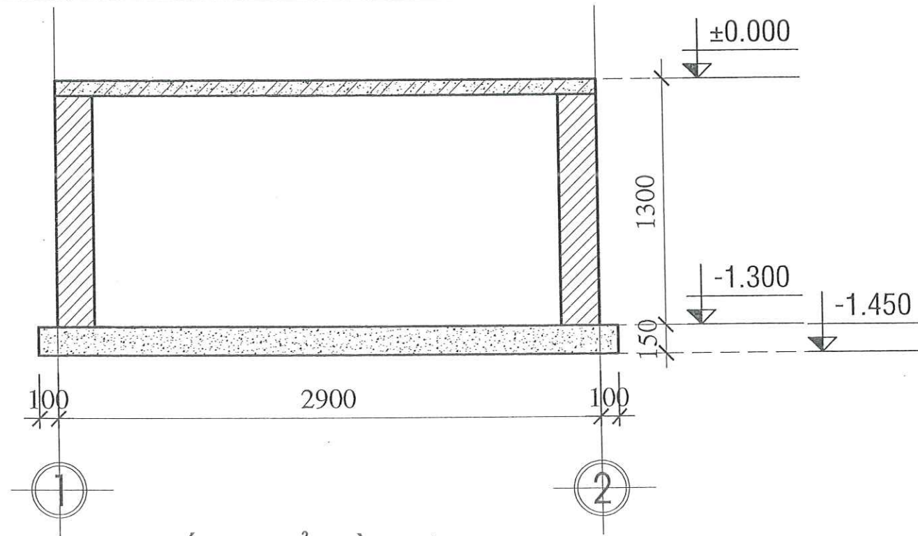
MẶT CẮT 1-1 BỂ ĐIỀU HOÀ TL 1/100
