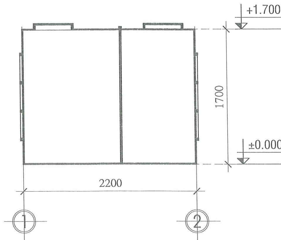
MẶT CẮT 1-1 TL 1/100
