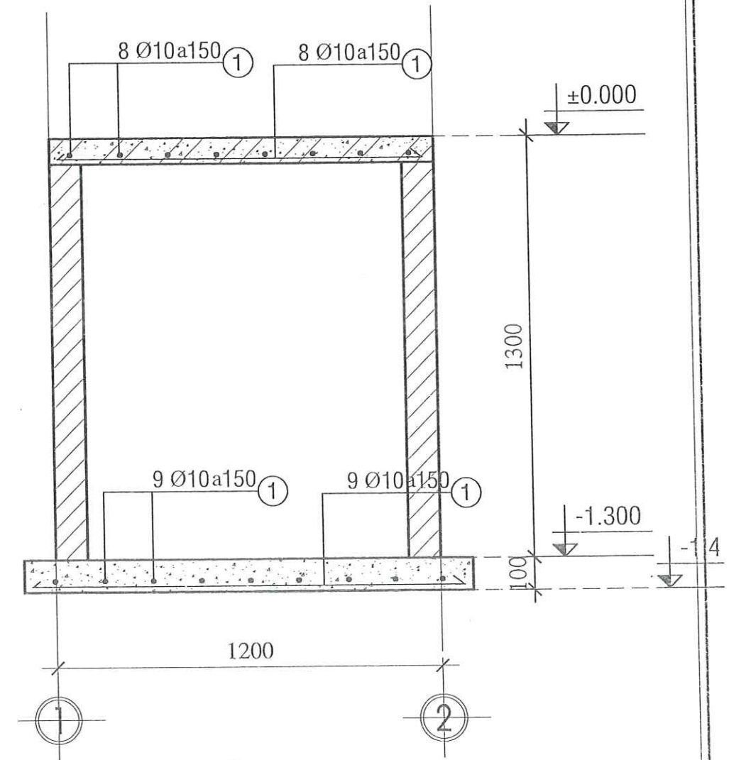
MẶT CẮT 1-1 HỒ GA TL 1/100
