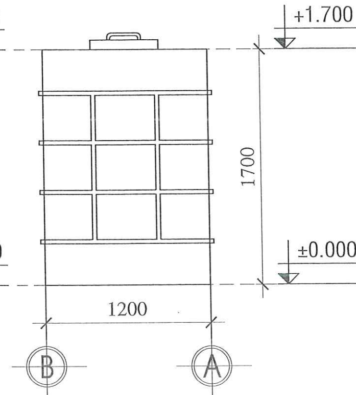
MẶT ĐỨNG TRỤC B-A TL 1/100
