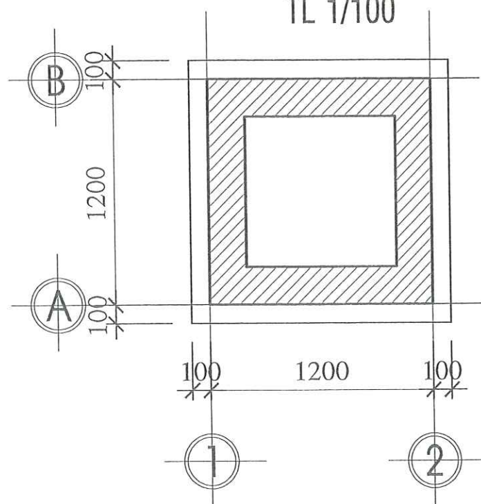
MẶT BẰNG BẢN ĐÁY HỒ GA TL 1/100
